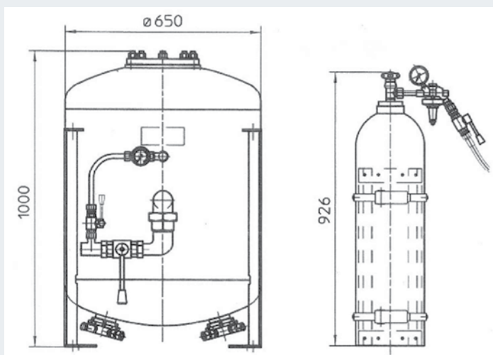
Slika 4. Ugradbene mjere sustava PLA 250
