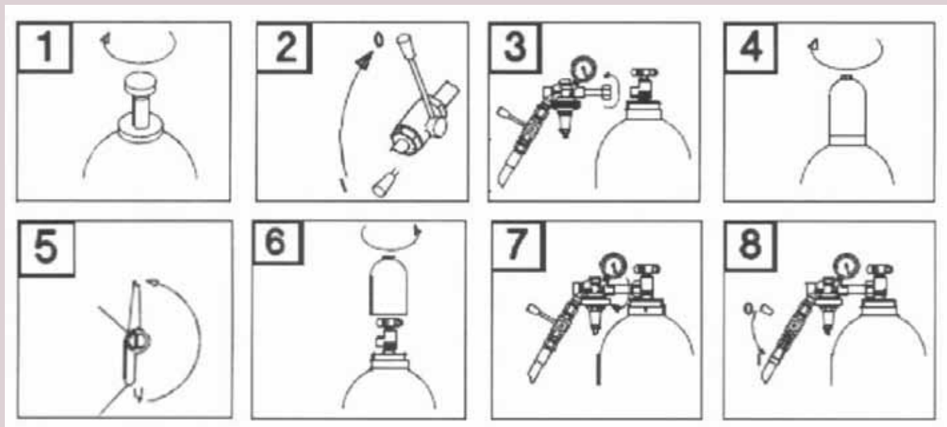
Slika 6. Slikovni prikaz redoslijeda radnji pri promjeni boce
